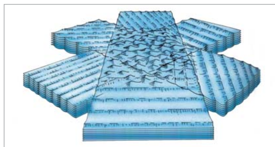
► Interne golven op grensvlak tussen twee lagen van water met verschillende dichtheden. De ene is zwaar (de onderste), de andere heeft een mindere dichtheid (de bovenste). (Oceanography, bruto, p. 204).
