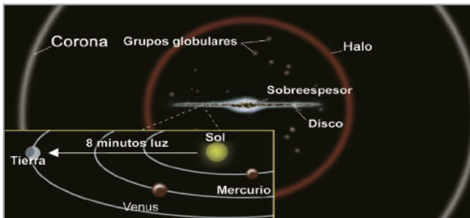
► Η εικόνα απεικονίζει τον γαλαξία μας και τους διαφορετικούς πλανήτες
