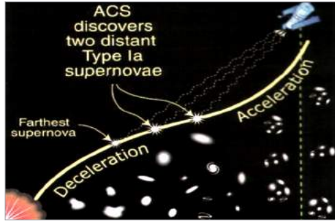
► Η εικόνα δείχνει ότι το σύμπαν διαστέλλεται.
