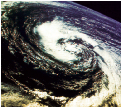
► Μια φωτογραφία της ατμόσφαιρας που συμπεριλαμβάνει τα σύννεφα και τους ανέμους της.
