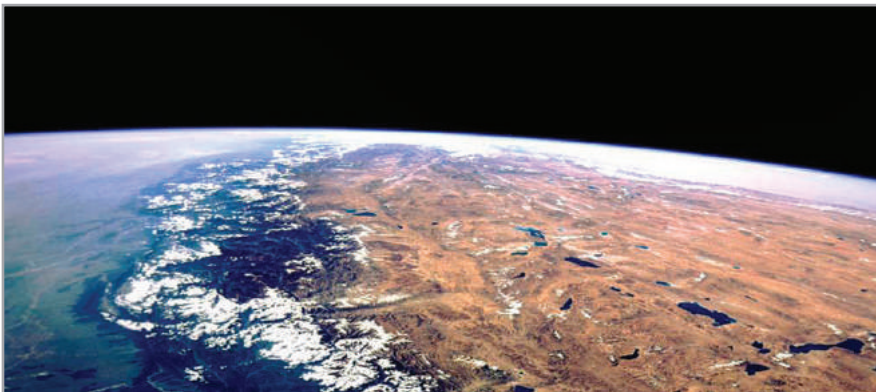
Diese Abbildung zeigt die Dünne des Tagesgürtels auf der Sonnenseite der Erde, der gerade 200km dick ist, wohingegen auf dem Rest der Erde absolute Dunkelheit herrscht.
