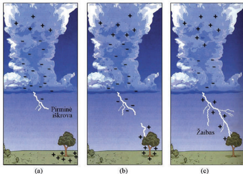
Antžeminio žaibo susidarymas. (a) Kai apatinėje debesies dalyje susikongruavęs neigiamas krūvis pasidaro pakankamai didelis, kad nugalėtų oro pasipriešinimą, susiformuoja pirminė debesies iškrova. (b) Jai priešpriešais, iškilnuose žemės taškuose, susikongruuoja teigiami krūviai – pirminė žemės iškrova. Šios dvi iškrovos beveik nematomos. (c) Kai debesies neigiamų krūvių srautas susiduria su žemės teigiamų krūvių srautu, srovė išauga kelis kartus ir trenkia antrinė iškrova – žaibas.
